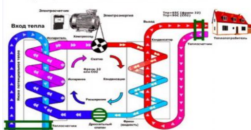
Принципиальная схема теплового насоса
